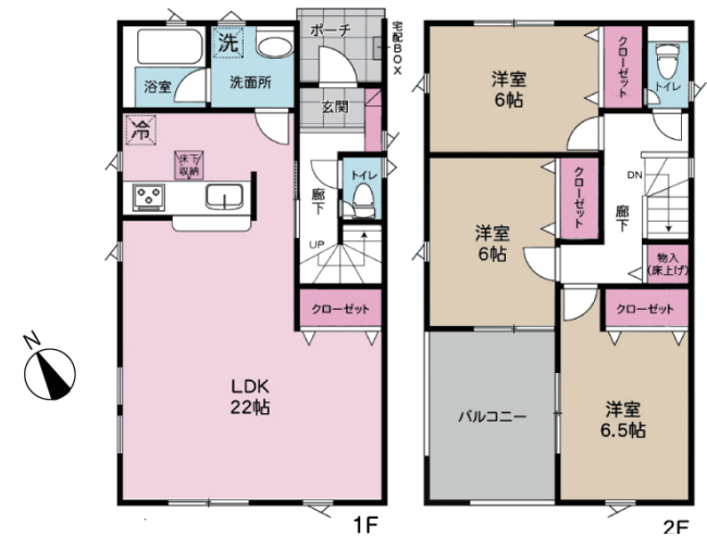
1号地間取図
