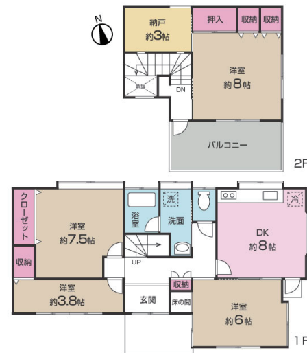
間取図
