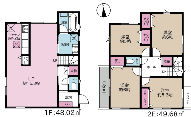
C号棟間取図
