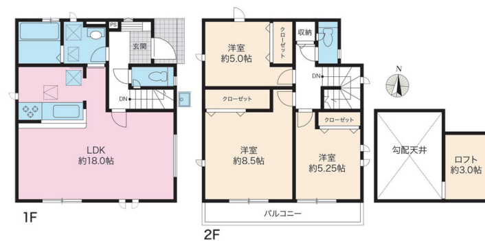
間取図
