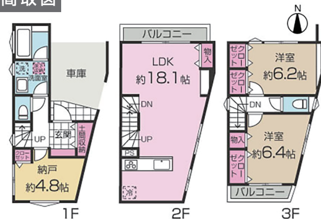
1号棟 間取図
