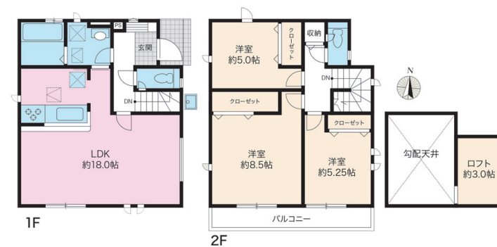
問取図
