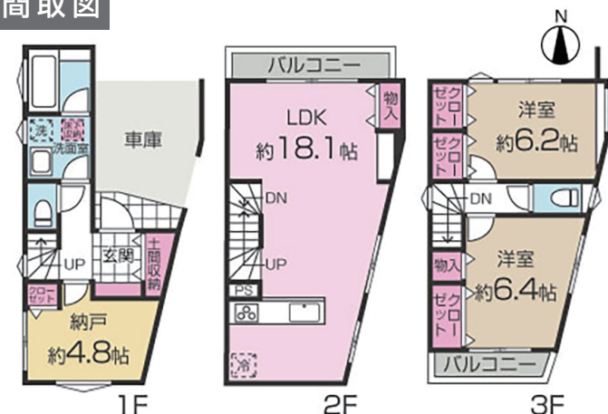
1号棟 間取図
