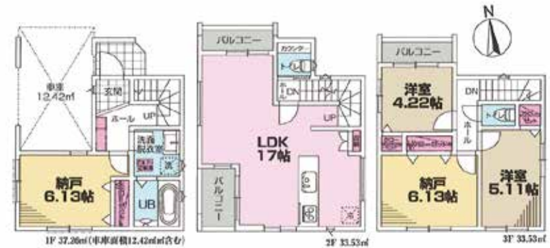
2号棟間取図
