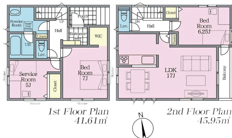
間取図
