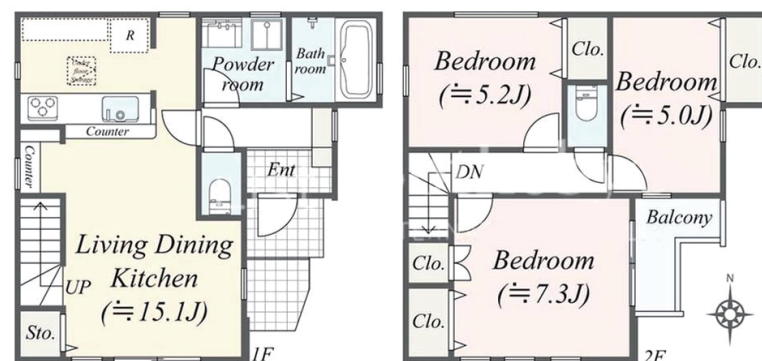
間取図
