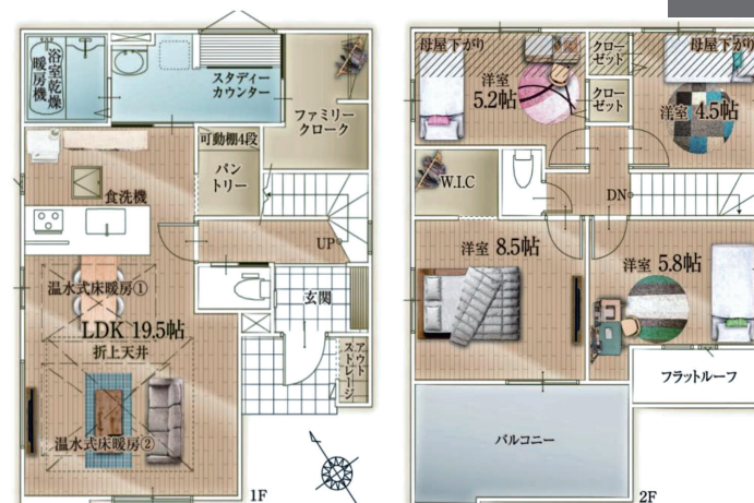
間取図
