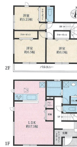
1号棟間取図
