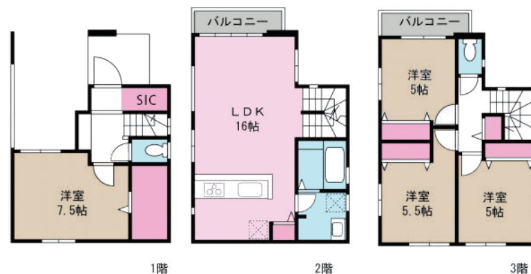
2号棟間取図
