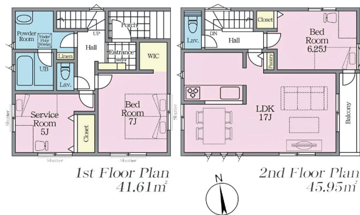
1号棟間取図
