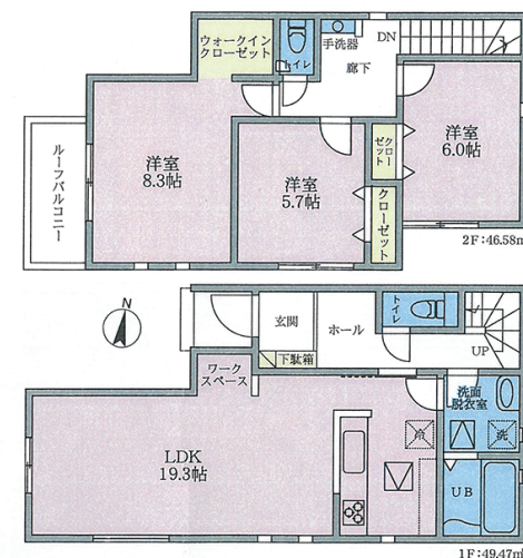
間取図
