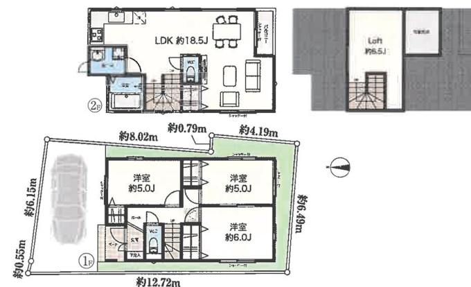
1号棟間取図
