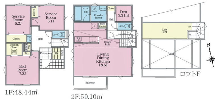
3号棟間取図
