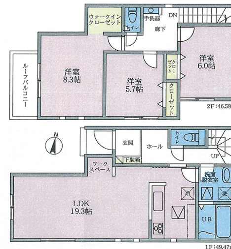
間取図
