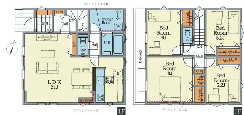
2号棟間取図
