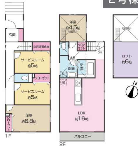
2号棟間取図
