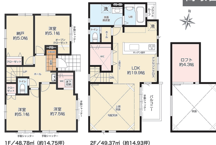
間取図
