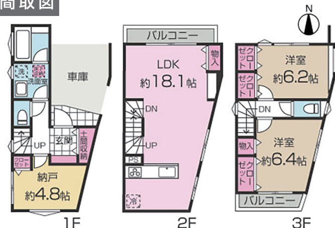
1号棟 間取図
